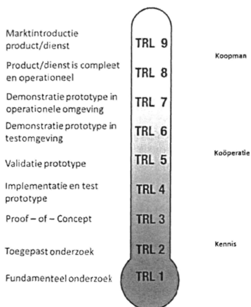
Figuur 1 TRL-model
